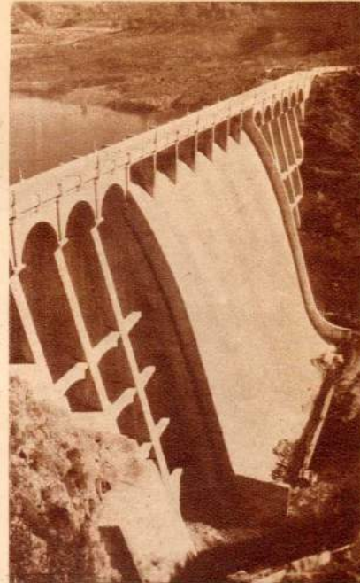
El dique Escaba, construido en la provincia de Tucumán, sobre el río Marapa, costó cincuenta millones de pesos y permite la irrigación de 29.500 hectáreas de tierra.
