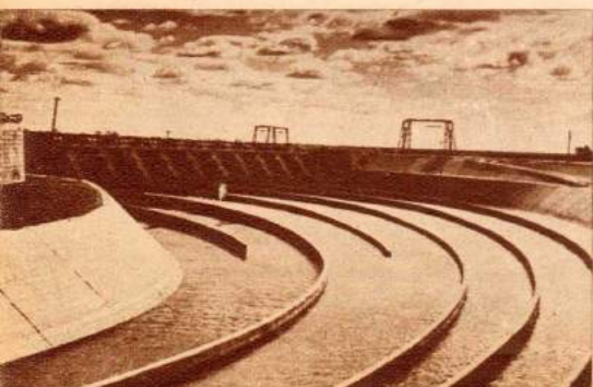
Un aspecto del dique Los Quiquinchos, construido por el gobierno del General Perón en la provincia de Santiago del Estero, cuyo costo alcanzó a la suma de $ 47.300.000.
