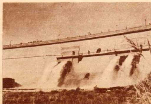
En los grabados que están en el centro y a la derecha pueden apreciarse dos aspectos del dique Nihuil, construido recientemente en Mendoza, y cuyo costo es de $ 6.500.000.
